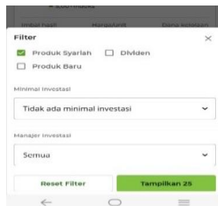
Gambar 3. Mengatur Filter.
