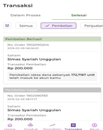
Gambar 6. Pembelian Berhasil.
